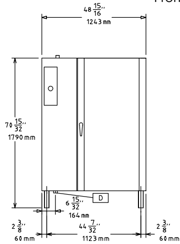
Front aanzicht
